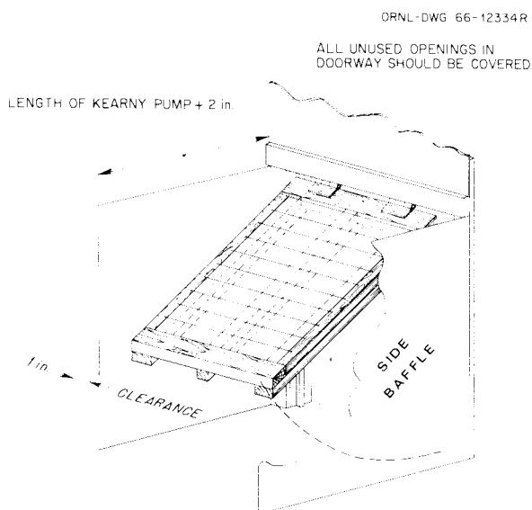
Fig. 25. Side baffles.
